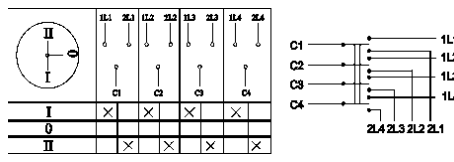
Пакетный переключатель ПП 4-полюсный на 2 направления
