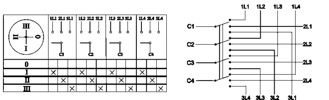
Пакетный переключатель ПП 4-полюсный на 3 направления
