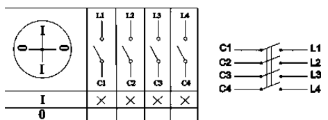
Пакетный выключатель ПВ 4-полюсный
