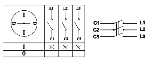
Пакетный выключатель ПВ 3-полюсный
