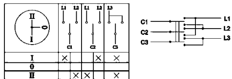
Пакетный переключатель ПП 3-полюсный реверсный
