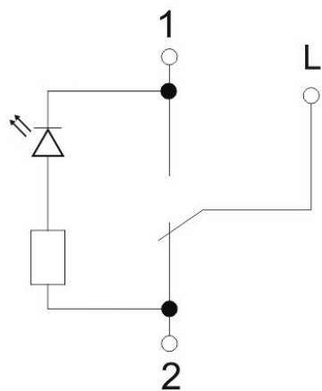
Рисунок 1 – Электрическая схема выключателя BS10-1-7-BrX*
