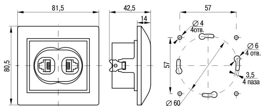
Рисунок 2. Розетки телефонные и компьютерные/телефонные РТ12-КБ, РТ12-ККм, РК/Т12-КБ, РК/Т12-ККм
