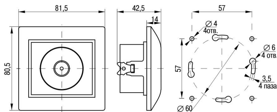
Рисунок 3. Розетки телевизионные РТВ10-КБ, РТВ10-ККм
