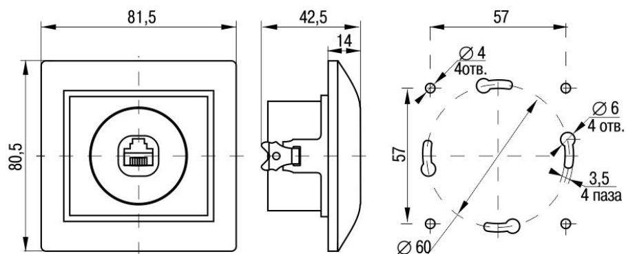
Рисунок 1. Розетки телефонные и компьютерные РТ10-КБ, РТ10-ККм, РК10-КБ, РК10-ККм
