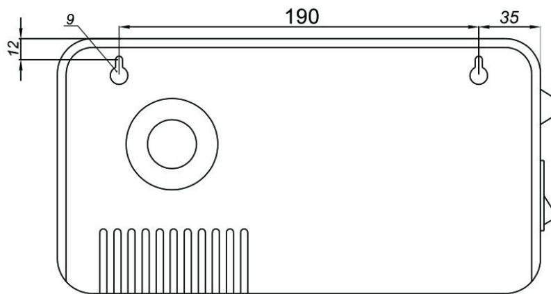
Рисунок 1. Верхняя панель стабилизатора
