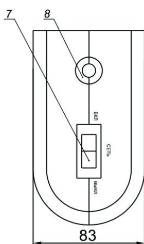
Рисунок 2. Левая боковая панель стабилизатора
