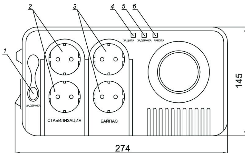
Рисунок 1. Верхняя панель стабилизатора
