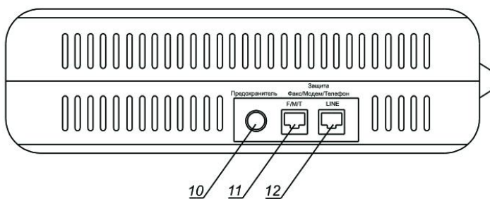
Рисунок 4. Задняя панель стабилизатора
