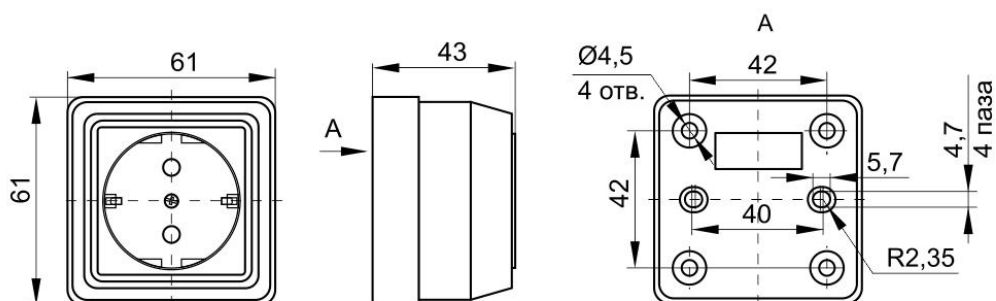
Рисунок 2. Розетки PC20-3-ОБ; PC20-3-ОКм; PC20-3-ОС; PC20-3-ОД; PCш20-3-ОБ; PCш20-3-ОКм; PCш20-3-ОС; PCш20-3-ОД.
