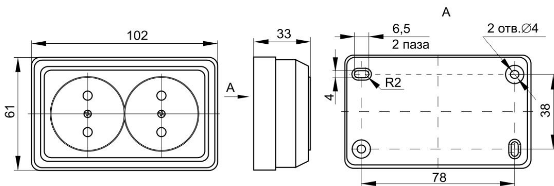
Рисунок 3. Розетки PC22-2-ОБ; PC22-2-ОКм; PC22-2-ОС; PC22-2-ОД; PCш22-2-ОБ; PCш22-2-ОКм; PCш22-2-ОС; PCш22-2-ОД.
