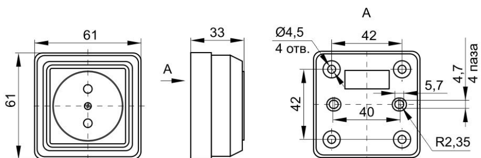
Рисунок 1. Розетки PC20-2-ОБ; PC20-2-ОКм; PC20-2-ОС; PC20-2-ОД; PCш20-2-ОБ; PCш20-2-ОКм; PCш20-2-ОС; PCш20-2-ОД.
