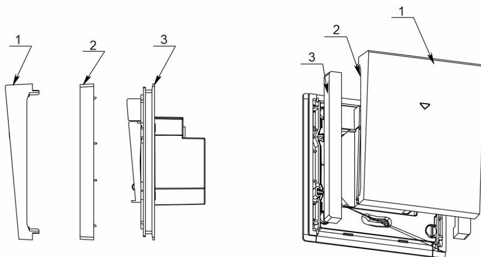
Рисунок 1 – Порядок монтажа выключателя
