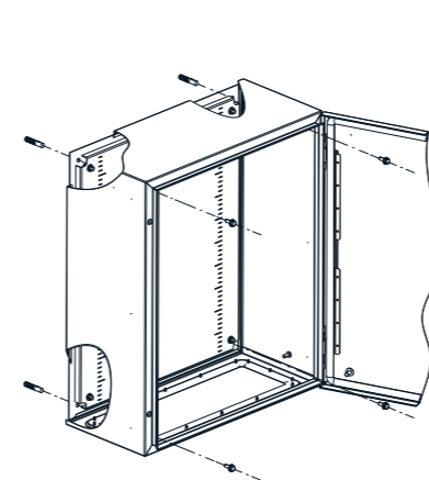
Монтаж к стене без зацепа
