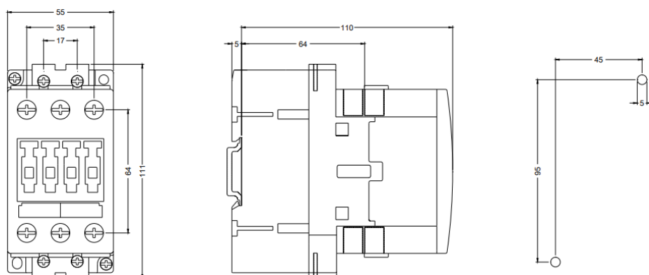
Габаритные размеры 3RT1034, 3RT1035, 3RT1036 с 3RH1921-1FA и 3RH1921-1EA
