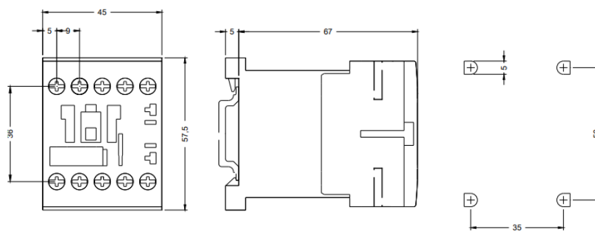
Габаритные размеры 3RT1015, 3RT1016, 3RT1017 с 3RH1911-1FA
