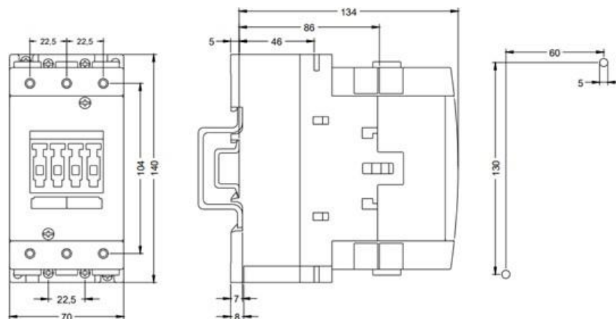
Габаритные размеры 3RT1044, 3RT1045, 3RT1046 с 3RH1921-1FA и 3RH1921-1EA
