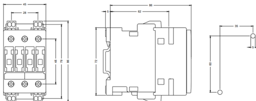
Габаритные размеры 3RT1023, 3RT1024, 3RT1025, 3RT1026 с 3RH1921-1FA и 3RH1921-1EA
