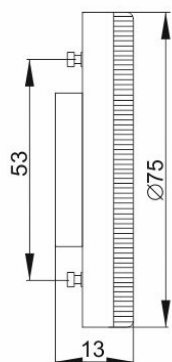
Рисунок 1 – Лампа LED-T75, 4 Вт, 6 Вт, 8 Вт, цоколь GX53
