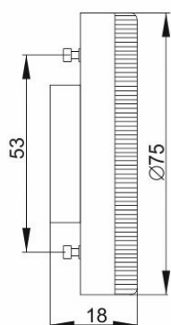
Рисунок 2 – Лампа LED-T75, 10 Вт, цоколь GX53
