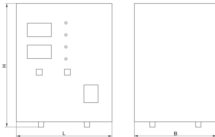
Рисунок 1 – Габаритные размеры:
