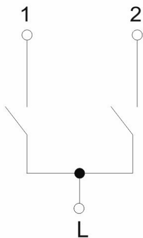
Рисунок 1 – Электрическая схема выключателей ВС10-2-0-БрХ*, ВСП10-2-0-БрХ*
