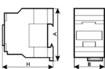
Рисунок 1. Контактор нереверсивный ПМЛ-1
