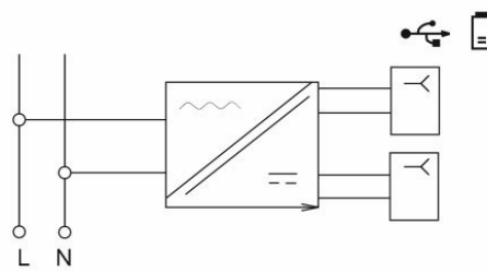
е) розетка / socket / prizele USB type A + type A
