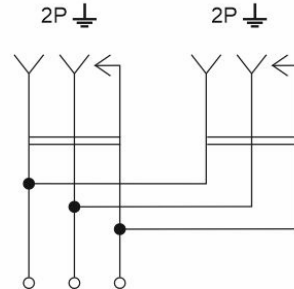
г) двухместная с заземлением
