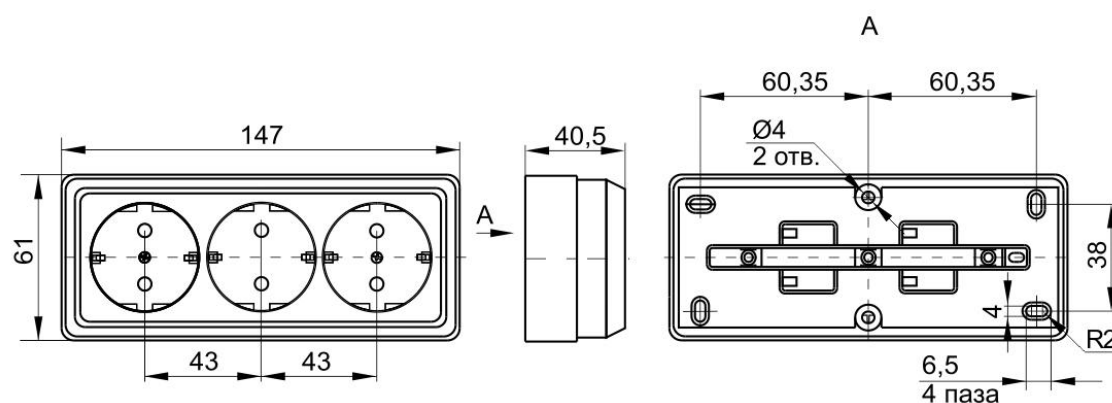
Рисунок 6. Розетки PC23-3-ОБ; PC23-3-ОК; PC23-3-ОС; PC23-3-ОД.
