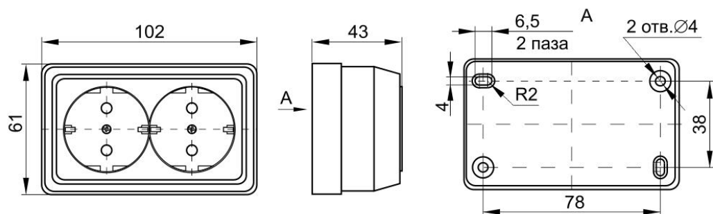
Рисунок 4. Розетки PC22-3-ОБ; PC22-3-ОКм; PC20-3-ОС; PC20-3-ОД; PCш20-3-ОБ; PCш20-3-ОКм; PCш20-3-ОС; PCш20-3-ОД.
