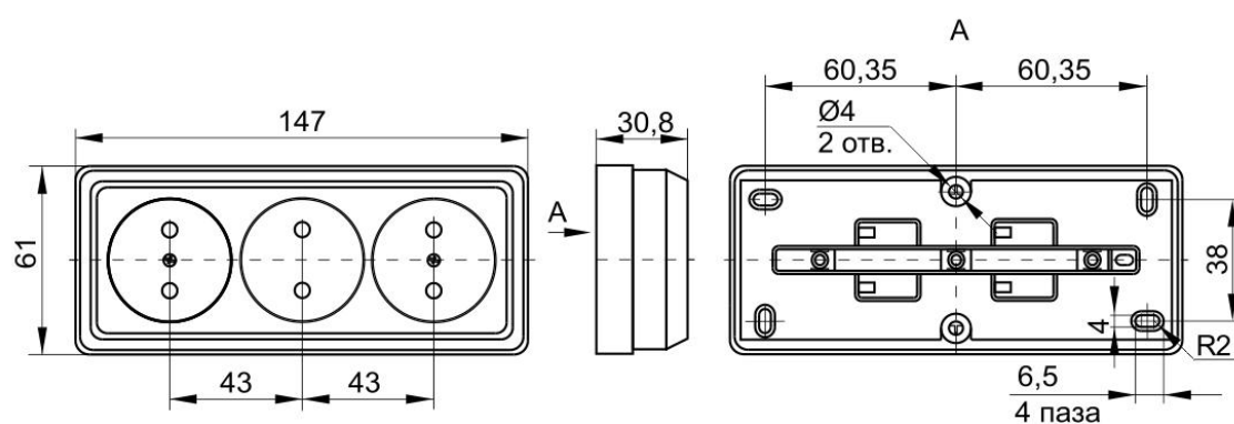
Рисунок 5. Розетки PC23-2-ОБ; PC23-2-ОК; PC23-2-ОС; PC23-2-ОД.
