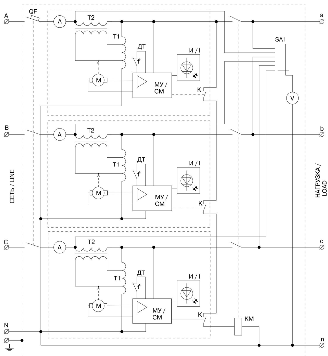
Рисунок 1б – Структурные схемы стабилизаторов: СНИЗ-15 кВА; СНИЗ-20 кВА; СНИЗ-30 кВА; СНИЗ-45 кВА; СНИЗ-60 кВА с дополнительным вольтодобавочным трансформатором
