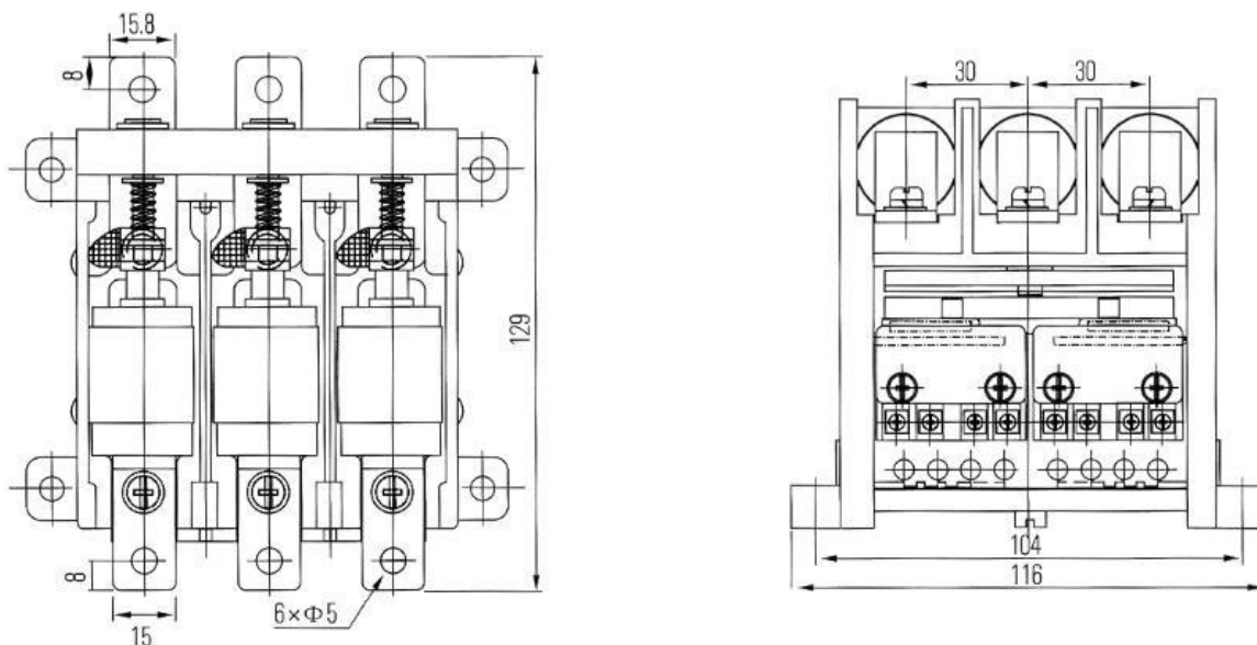
Рисунок 1. Габаритные размеры КВТ-1,14-63
