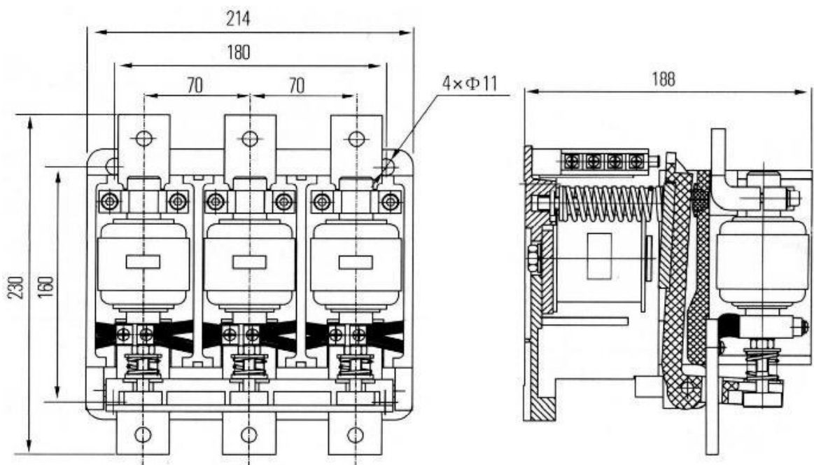
Рисунок 4. Габаритные размеры КВТ-1,14-400
