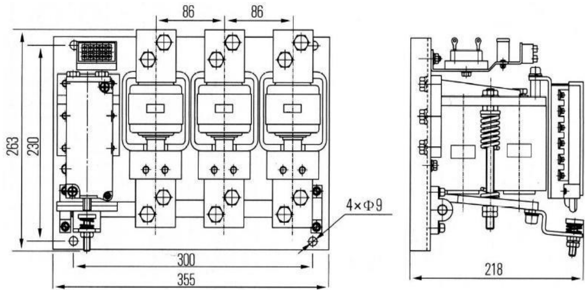
Рисунок 5. Габаритные размеры КВТ-1,14-630
