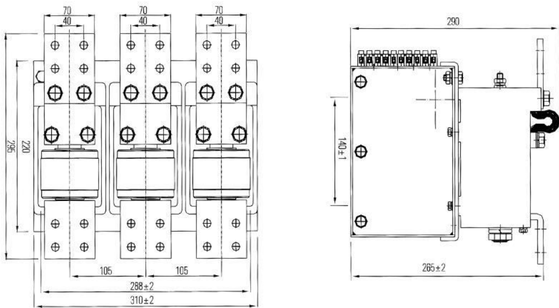
Рисунок 6. Габаритные размеры КВТ-1,14-1000/1250
