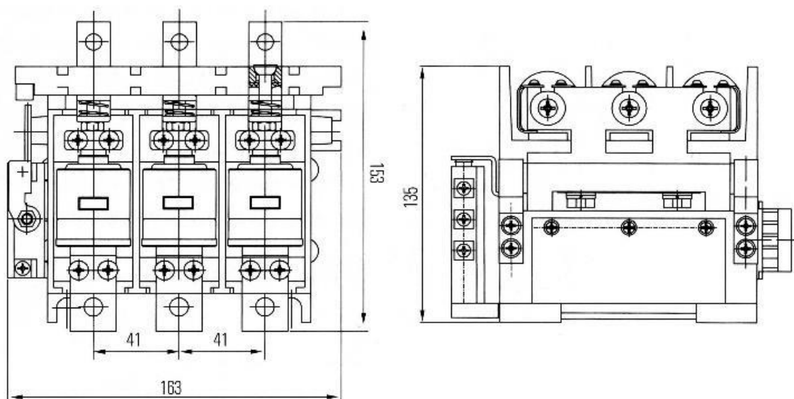
Рисунок 2. Габаритные размеры КВТ-1,14-80/125/160
