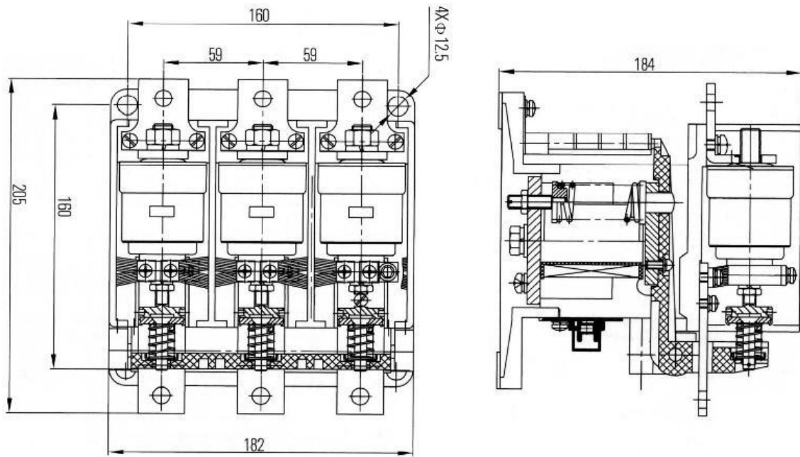
Рисунок 3. Габаритные размеры КВТ-1,14-250
