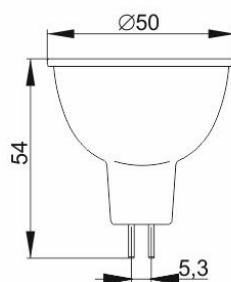
Рисунок 3 – Лампа LED–MR16, 9 Вт цоколь GU5.3
