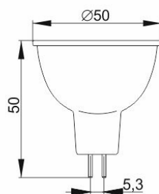
Рисунок 2 – Лампа LED–MR16, 7 Вт цоколь GU5.3
