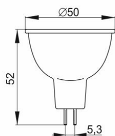
Рисунок 1 – Лампа LED–MR16, 3 Вт, 5 Вт цоколь GU5.3
