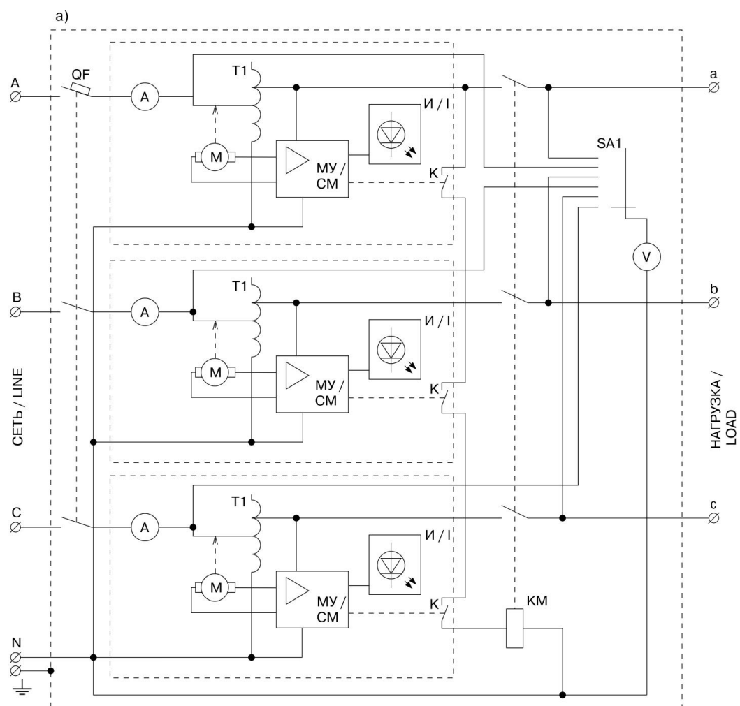
Рисунок 1а – Структурные схемы стабилизаторов: СНИЗ-3 кВА; СНИЗ-6 кВА; СНИЗ-7,5 кВА
