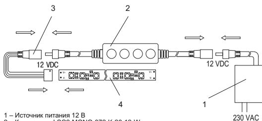
Рисунок 3 – Схема параллельного подключения одноцветной светодиодной ленты к блоку питания и контроллеру MONO (диммеру)
