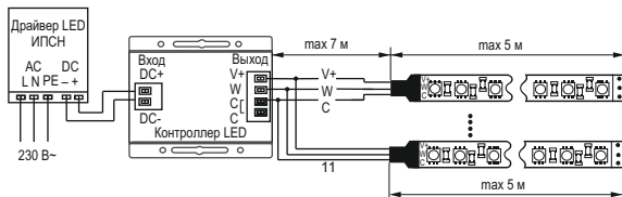
Рисунок 7 – Схема параллельного подключения мультibelой светодиодной ленты к блоку питания и контроллеру
