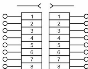
г) розетка компьютерная
