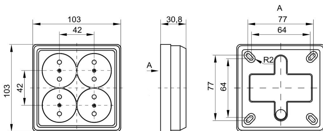
Рисунок 7. Розетки PC24-2-ОБ; PC24-2-ОК; PC24-2-ОС; PC24-2-ОД.
