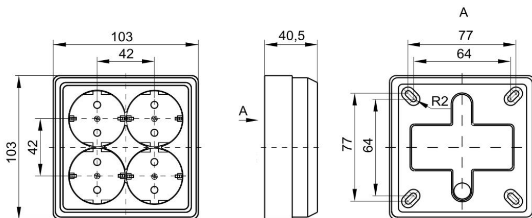
Рисунок 8. Розетки PC24-3-ОБ; PC24-3-ОК; PC24-3-ОС; PC24-3-ОД.
