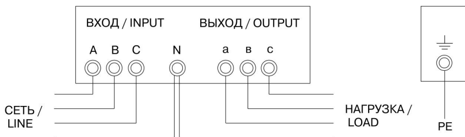
Рисунок 1 – Схема подключения СНИЗ-3 кВА
